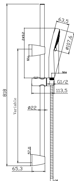
Артикул: 63068 Душевой гарнитур Neno (стойка) 5 режимов шланг 200 PVC
