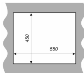
УСТАНОВОЧНЫЙ ПРОЁМ
