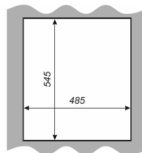
УСТАНОВОЧНЫЙ ПРОЁМ
