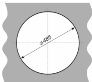
УСТАНОВОЧНЫЙ ПРОЁМ
