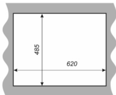
УСТАНОВОЧНЫЙ ПРОЁМ
