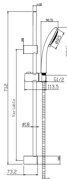
Артикул: 63067 Душевой гарнитур Vibe (стойка) 3 режима
