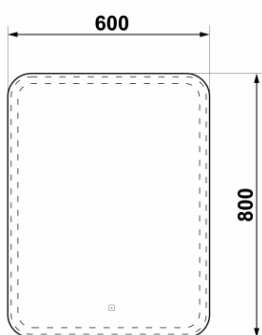
Зеркало-шкаф Cielo Led 600x800 правый, левый с розеткой, сенсорное вкл. A - 600 мм B - 800 мм C - 150 мм
