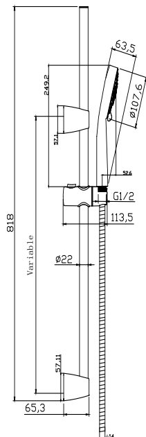
Артикул: 63068 Душевой гарнитур Neno (стойка) 5 режимов
